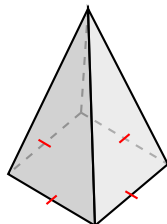
pirámide cuadrada
