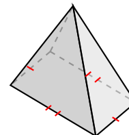
pirámide rectangular
