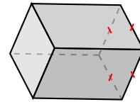
prisma cuadrado
