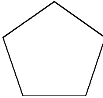
Pentágono Regular
