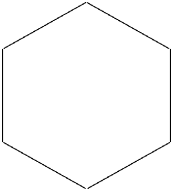
Hexágono Regular
