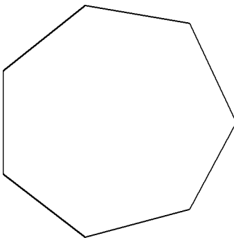
Heptágono Regular
