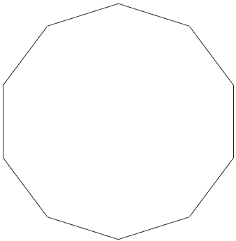
Decágono Regular
