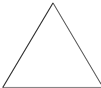
Triángulo Isósceles
