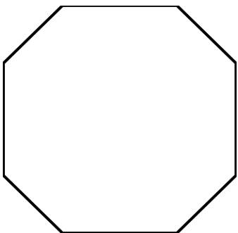
Octágono Regular
